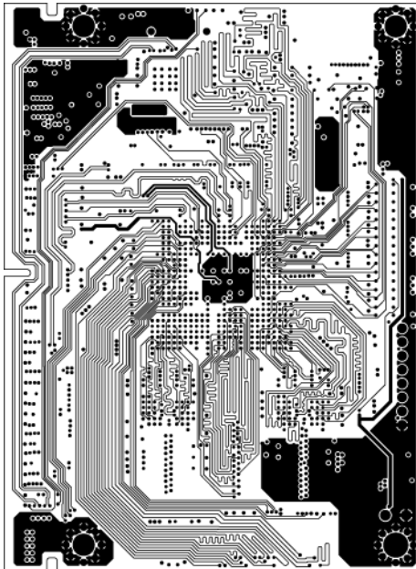
Layer 3: IN1
