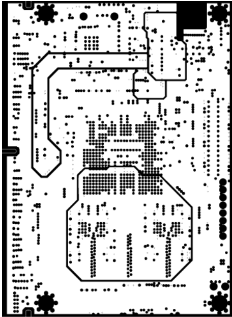
Layer 5: VCC2
