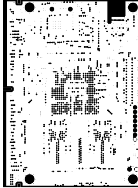
Layer 2: GND
