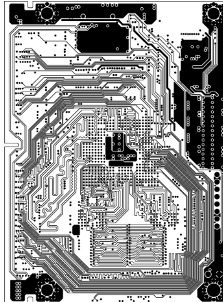
Layer 6: IN2
