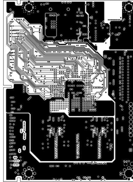
layer 4: VCC
