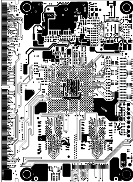
Layer 1: Top side
