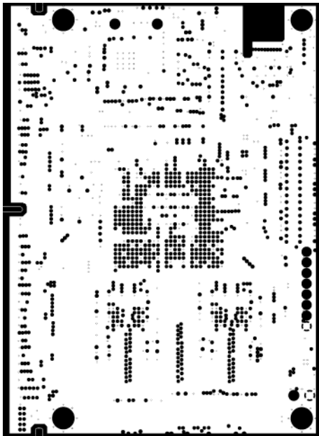
Layer 7: GND2
