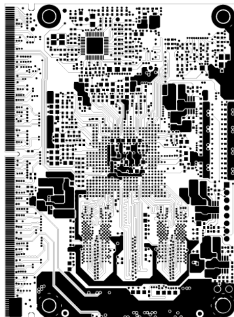
Layer 8: Bottom side
